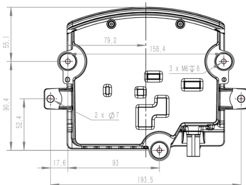
底视图
